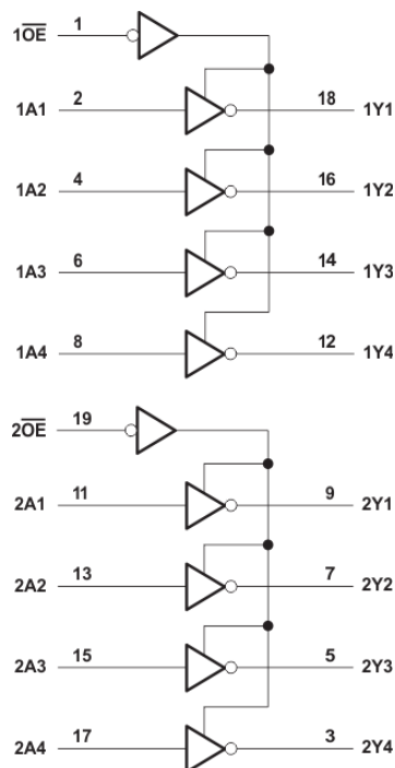
論理図 (正論理)
