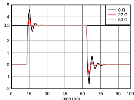
図 8-2. スwitching特性の比較
