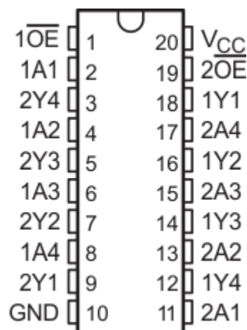
図 4-1. SN74LV8T240 PW または DGS パッケージ、20 ピン TSSOP または VSSOP (上面図)
