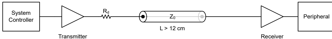
図 10-1. 代表的なアプリケーションのブロック図
