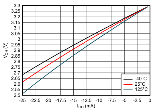
図 5-18. High 状態における出力電圧と電流との関係、3.3V 電源
