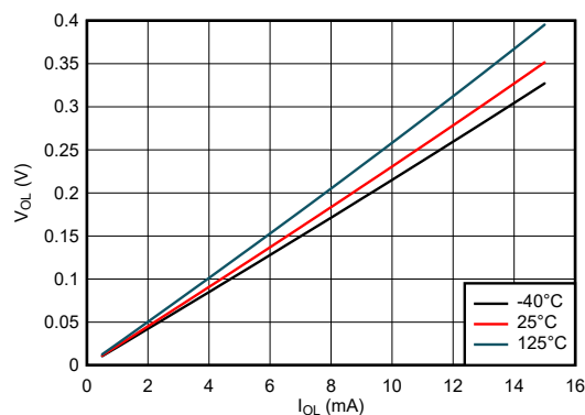
図 5-21. Low 状態における出力電圧と電流との関係、2.5V 電源
