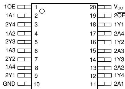
図 4-1. PW または DGS パッケージ、20 ピン TSSOP または VSSOP (上面図)
