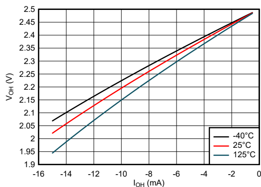
図 5-20. High 状態における出力電圧と電流との関係、2.5V 電源
