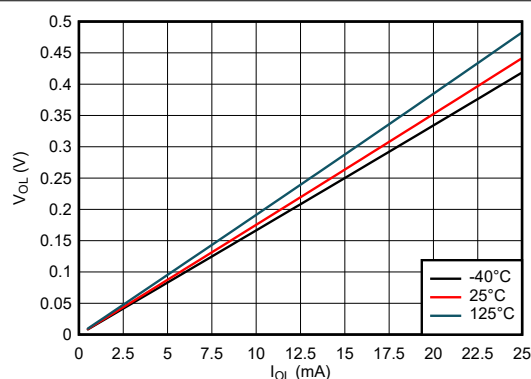
図 5-17. Low 状態における出力電圧と電流との関係、5V 電源
