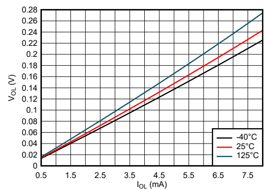
図 5-23. Low 状態における出力電圧と電流との関係、1.8V 電源
