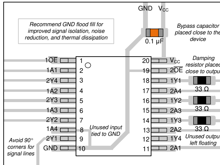
図 10-3. TSSOP の SN74LV8T244 のレイアウト例
