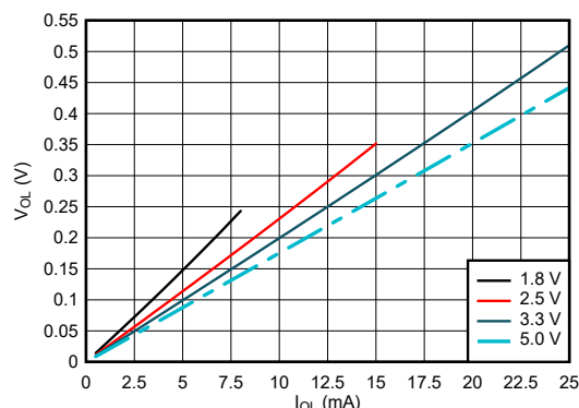
図 5-15. Low 状態における出力電圧と電流との関係
