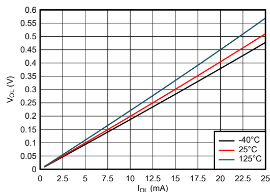
図 5-19. Low 状態における出力電圧と電流との関係、3.3V 電源
