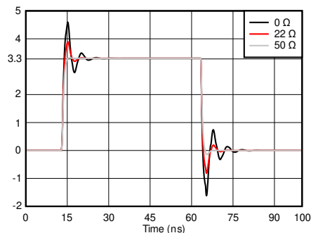
図 10-2. 異なるダンピング抵抗 ( R_d ) 値を使用してレシーバでのシグナル インテグリティをシミュレート
