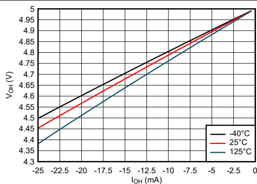
図 5-16. High 状態における出力電圧と電流との関係、5V 電源
