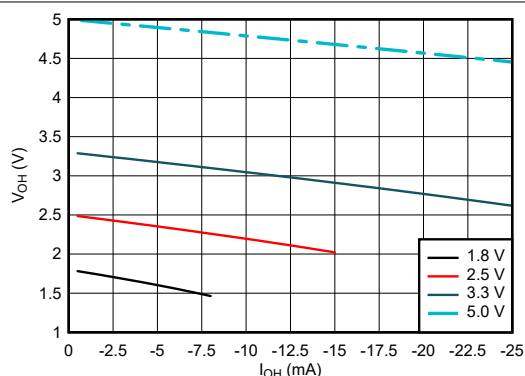
図 5-14. High 状態における出力電圧と電流との関係
