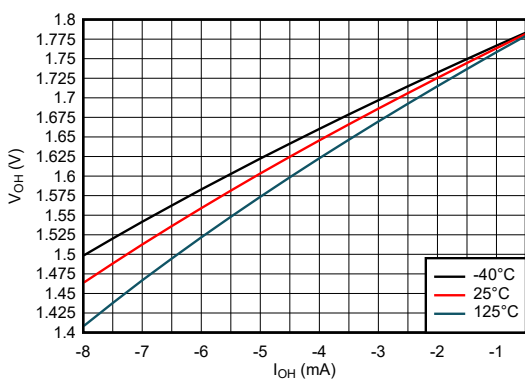
図 5-22. High 状態における出力電圧と電流との関係、1.8V 電源
