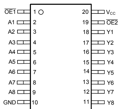
図 4-2. SN74LV8T540-Q1 PW、DGS パッケージ (上面図)
