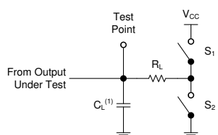
図 6-1.3 ステート出力の負荷回路
