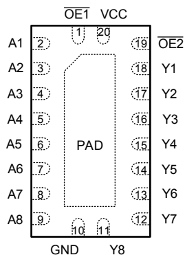
図 4-1. SN74LV8T541-Q1 RKS パッケージ (上面図)
