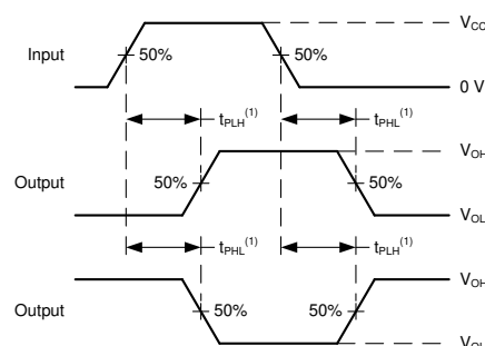
図 6-2. 電圧波形、伝搬遅延
