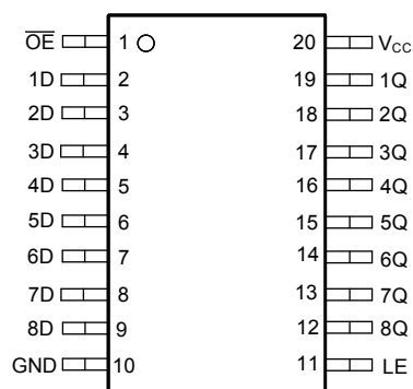
図 4-2. SN74LV8T573 PW、DGS パッケージ (上面図)
