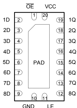
図 4-1. SN74LV8T573 RKS パッケージ (上面図)
