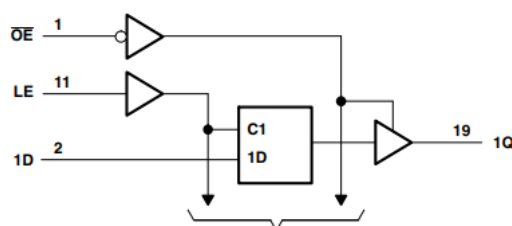
図 7-1. 7 個の他チャネルへの論理図 (正論理)
