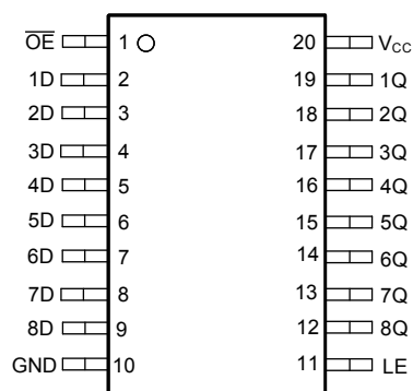
図 4-2. SN74LV8T573-Q1 PW、DGS パッケージ (上面図)
