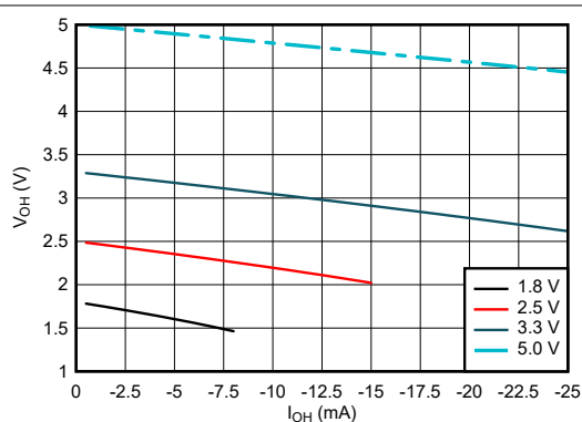
図 5-1. High 状態における出力電圧と電流との関係
