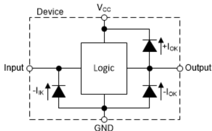
図 7-5. 各入力と出力に対するクランプ ダイオードの電氣的配置
