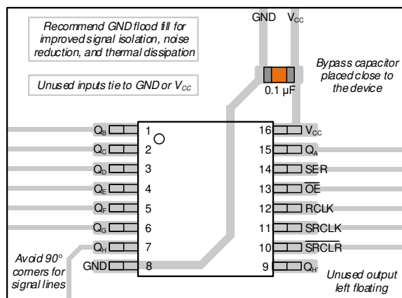
図 8-3. TSSOP の SN74LV8T596-Q1 のレイアウト例
