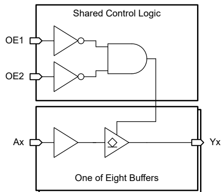
図 7-1. 論理図 (正論理)
