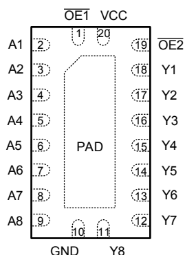
図 4-1. SN74LV8T7541 RKS パッケージ (上面図)
