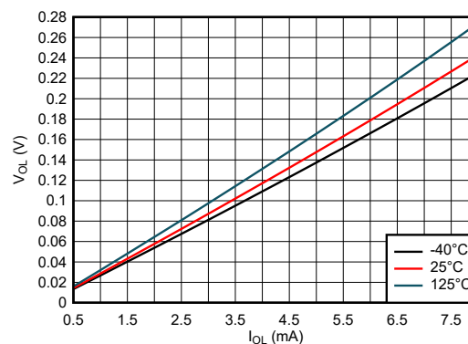
図 5-8. Low 状態における出力電圧と電流との関係、1.8V 電源
