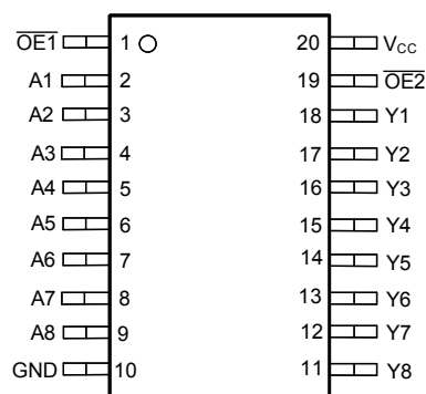
図 4-2. SN74LV8T7541 PW、DGS パッケージ (上面図)
