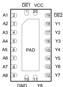
図 4-1. SN74LV8T7541-Q1 RKS パッケージ (上面図)
