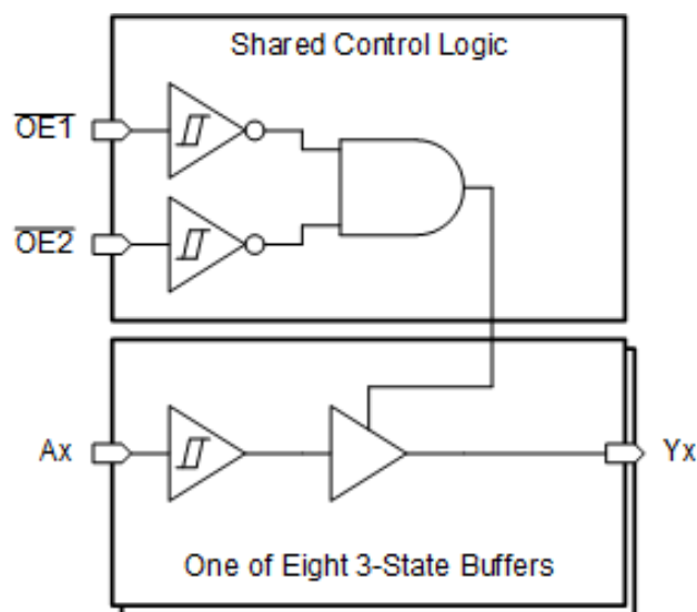
論理図 (正論理)
