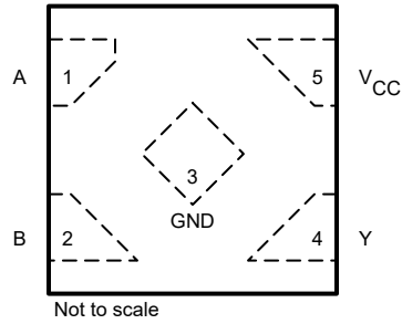
図 4-1. DTX パッケージ、5 ピン X2SON (上面図)
