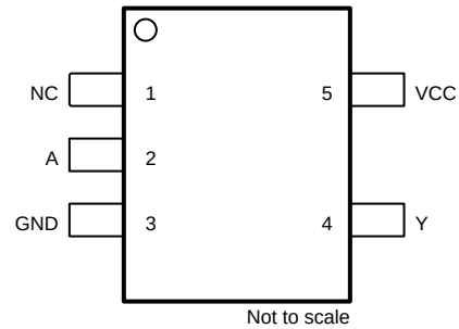
図 4-2. SN74LVC1G37-Q1 DCK パッケージ、5 ピン SOT-SC70 (上面図)
