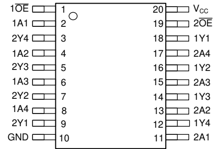
図 4-2. SN74LVC240A-Q1 PW、DGS パッケージ (上面図)
