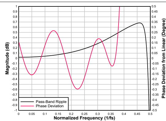
図 6-43. 低レイテンシ デシメーション フィルタのパスバンド リップルと位相偏差
