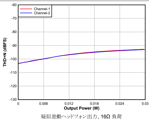
図 5-24. DAC THD+N レベルと出力電力との関係
