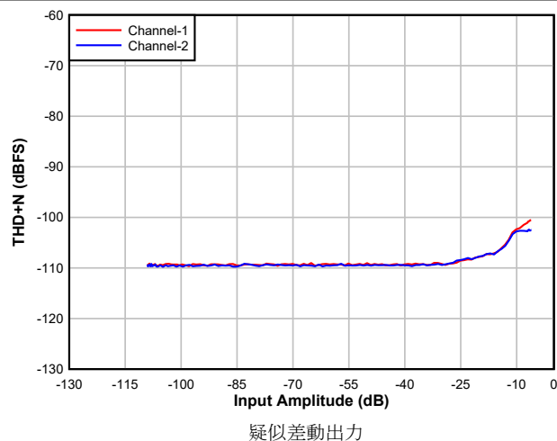
図 5-21. DAC の THD +N レベルと入力との関係
