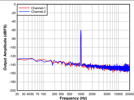
図 8-7. -60dBFS 入力の DAC FFT
