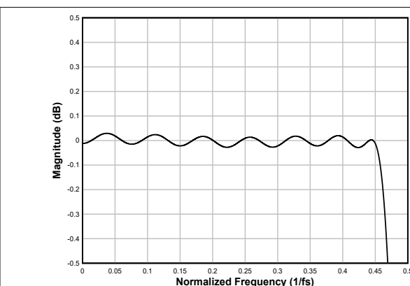
図 6-72. 線形位相補間フィルタのパスバンド リップル
