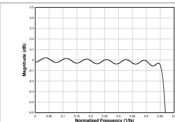
図 6-74. 線形位相補間フィルタのパスバンド リップル
