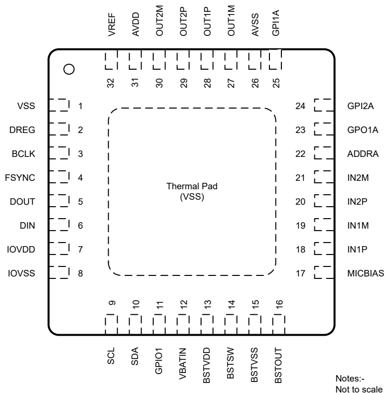
図 4-1. TAC5312-Q1 パッケージ、32 ピン WQFN (露出サーマル パッド付き) 上面図
