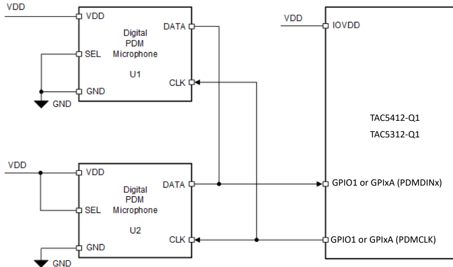
図 6-19. TAC5312-Q1 のデジタル PDM マイクの接続図
