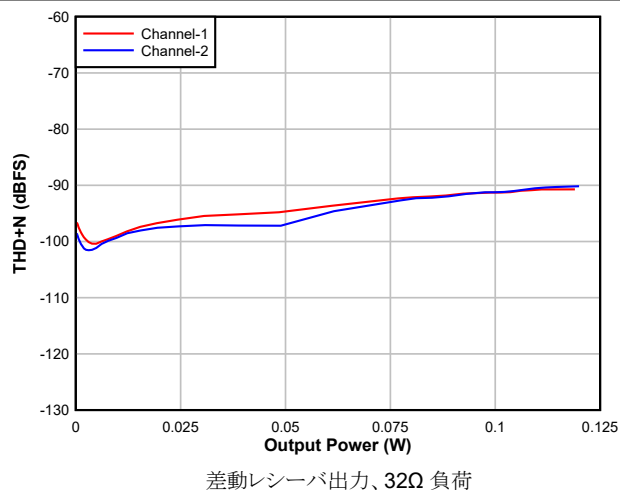
図 5-22. DAC THD+N レベルと出力電力との関係
