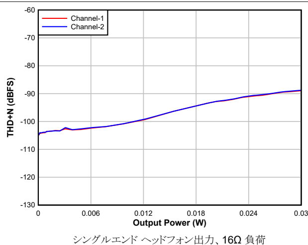
図 5-23. DAC THD+N レベルと出力電力との関係
