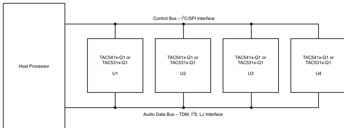
図 6-14. 制御およびオーディオ データ バスを共有する複数の TAC5312-Q1 デバイス
