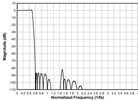
図 6-80. 低レイテンシのデシメーション フィルタの振幅応答
