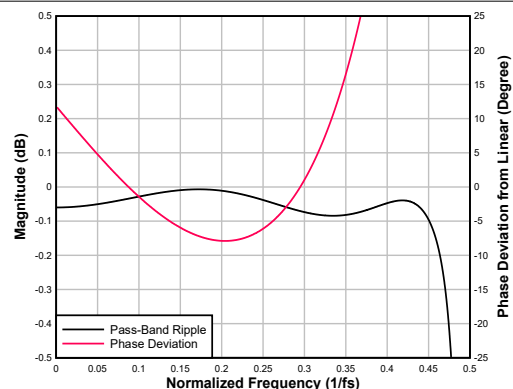
図 6-53. 超低レイテンシ補間フィルタのパスバンドリップルと位相偏差
