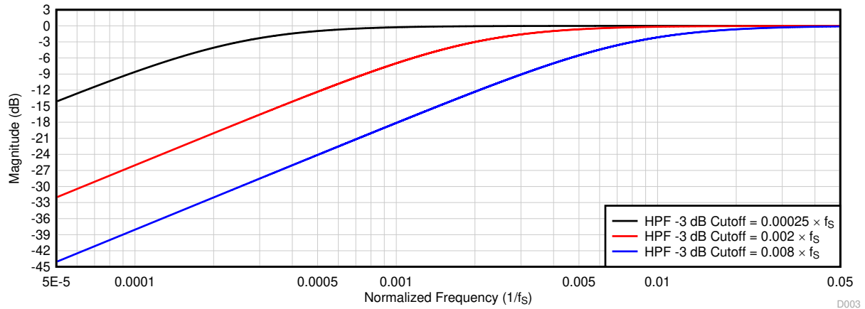
図 6-61. HPF フィルタの周波数応答プロット
