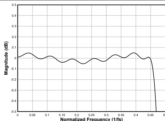
図 6-71. 線形位相デシメーション フィルタのパスバンド リップル
