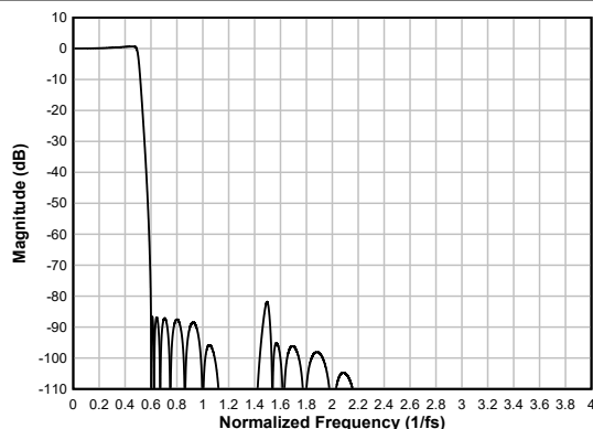
図 6-82. 低レイテンシのデシメーション フィルタの振幅応答
