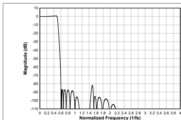
図 6-92. 超低レイテンシのデシメーション フィルタの 振幅応答
