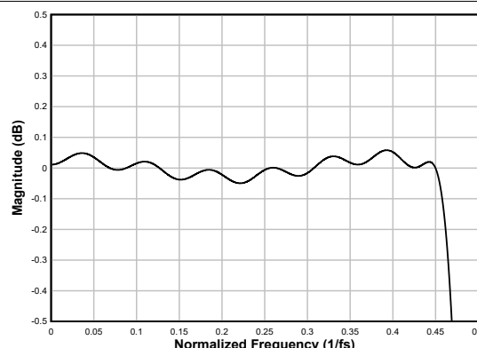
図 6-73. 線形位相デシメーション フィルタのパスバンド リップル
