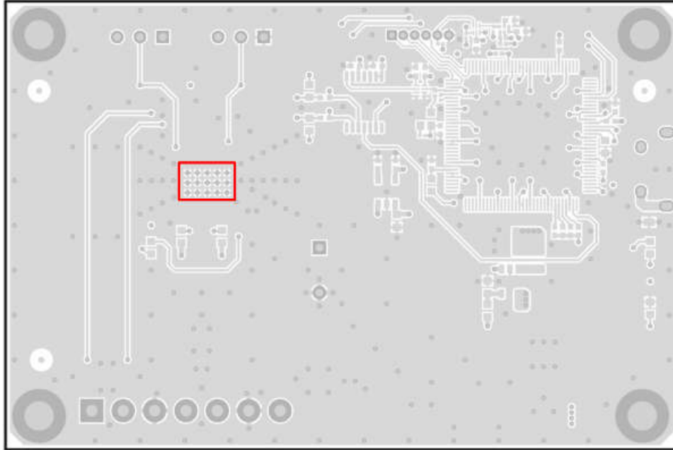
図 10-4. Bottom Layer
