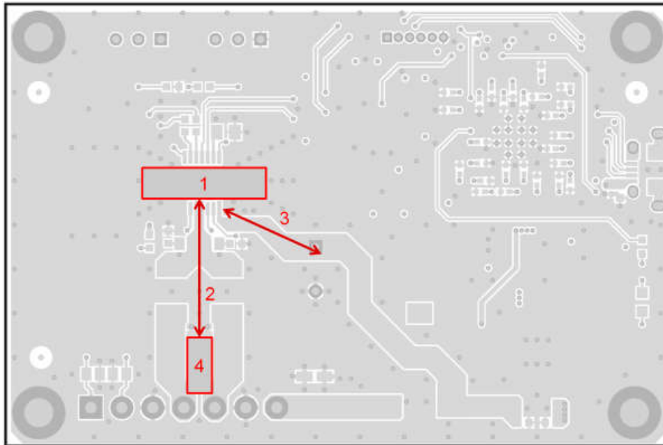
☒ 10-1. Top layer
