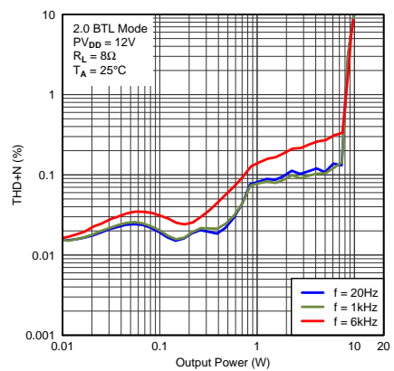
图 16. THD+N vs Output Power
