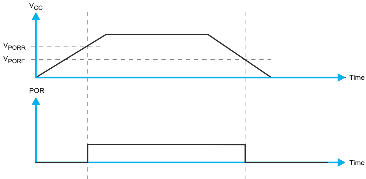
図 8-7. V_{POR}
