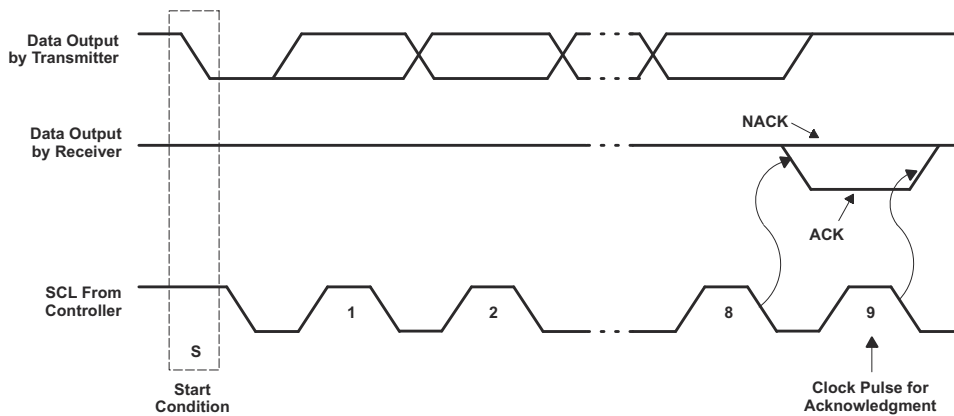
図 7-6. I 2 C バスのアクリッジ
