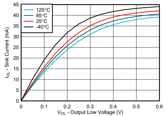
図 5-6. I/O シンク電流と出力 Low 電圧との関係、V CCP = 1.08V
