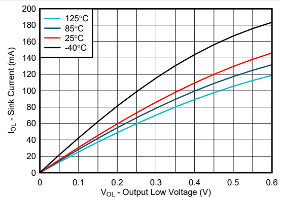
図 5-8. I/O シンク電流と出力 Low 電圧との関係、V CCP = 1.8V
