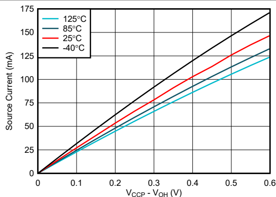
図 5-16. I/O ソース電流と出力 High 電圧との関係、 V CCP = 2.5V
