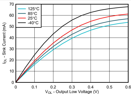
図 5-7. I/O シンク電流と出力 Low 電圧との関係、V CCP = 1.2V
