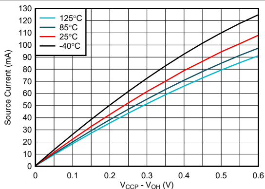
図 5-15. I/O ソース電流と出力 High 電圧との関係、 V CCP = 1.8V
