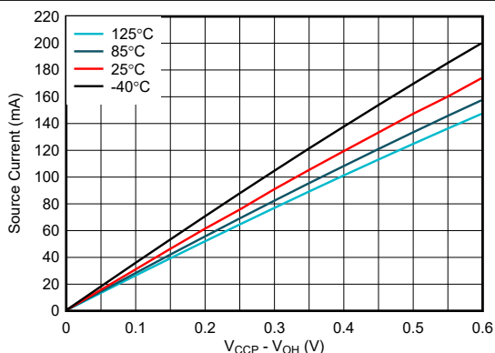
図 5-17. I/O ソース電流と出力 High 電圧との関係、 V CCP = 3.3V
