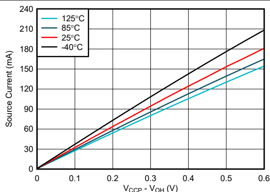
図 5-18. I/O ソース電流と出力 High 電圧との関係、 V CCP = 3.6V
