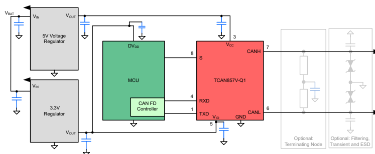
概略回路図
