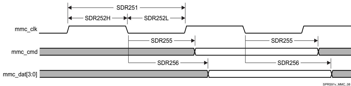
図 7-46. MMC/SD/SDIOj in - SDR25 - Transmitter Mode
