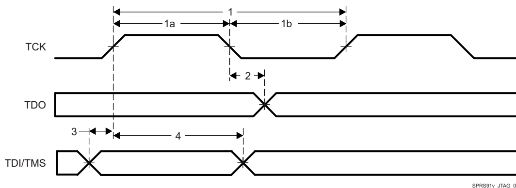
图 7-47. JTAG Timing
