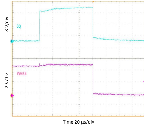
图 27. IO-Link WAKE, Low Side Mode
