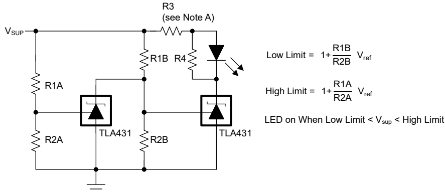
図 9-8. 電圧モニタ
