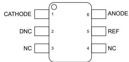
図 5-3. DRL パッケージ、 6 ピン SOT-563、TLA431 (上面図)
