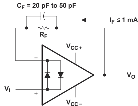
図 8-1. 電圧フォロワ
