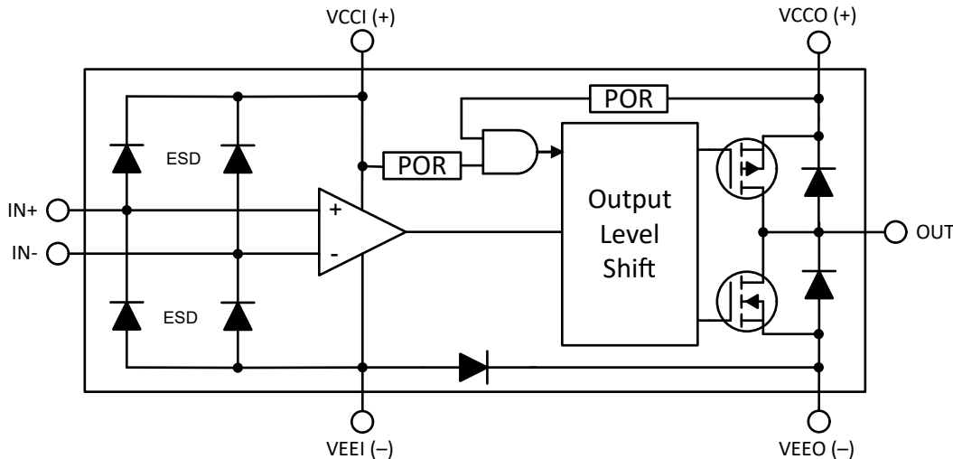
図 6-1. Block Diagram
