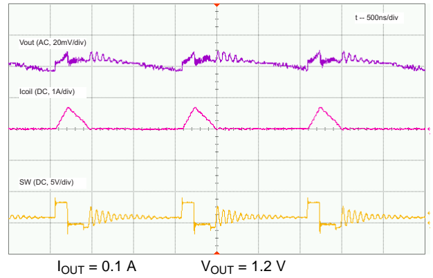
FIG 12. PFM Operation
