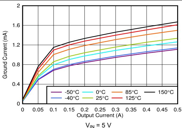
图 6-6. I_{GD} vs I_{OUT}
