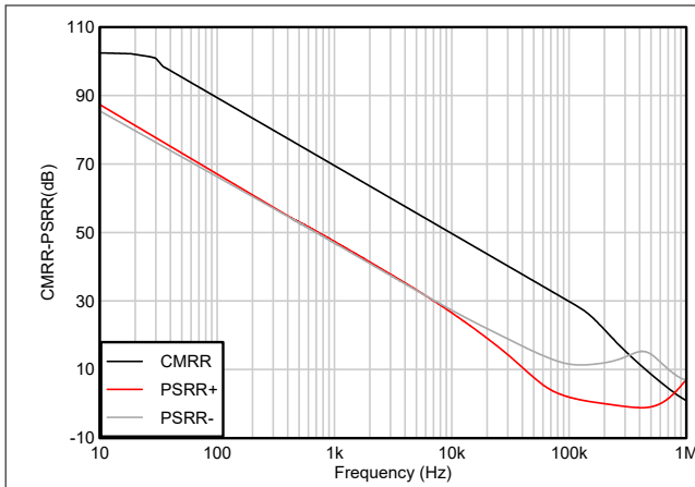
図 5-7. CMRR and PSRR vs Frequency
