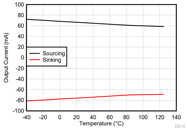
図 6-38. 短絡電流と温度との関係
