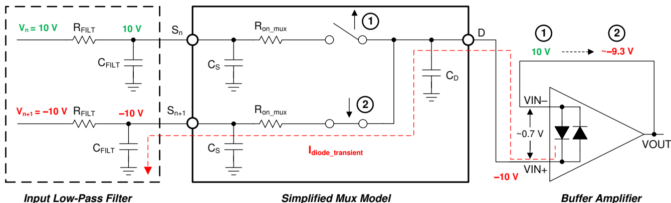
図 7-2. バック・ツー・バック・ダイオードではセtringの問題が発生する
