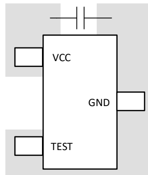
図 11-1. TMAG5124-Q1 Layout Example
