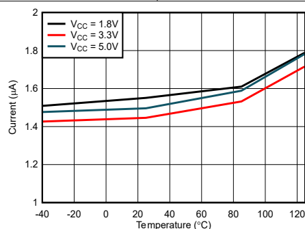
図 6-7. 20Hz I_{CCAVG} と温度との関係
