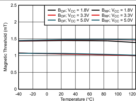
図 6-3. 1.5mT B_{OP} および B_{RP} スレッシュホールドと温度との関係
