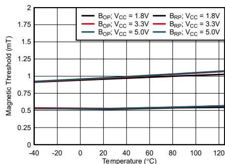
図 6-1. 1.0mT B_{OP} および B_{RP} スレッシュホールドと温度との関係
