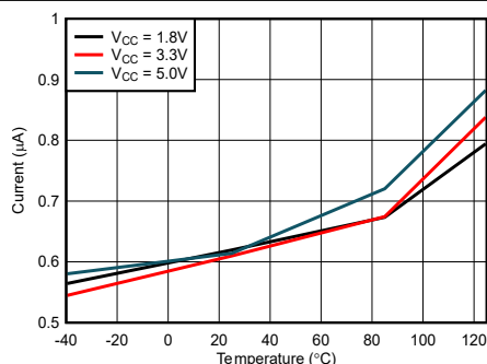
図 6-5. 5Hz I_{CCAVG} と温度との関係
