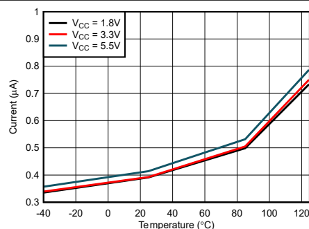
図 6-4. 1.25Hz I_{CCAVG} と温度との関係
