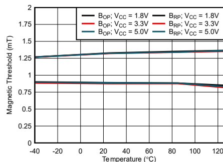
図 6-2. 1.3mT B_{OP} および B_{RP} スレッシュホールドと温度との関係
