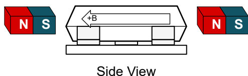
図 7-3. 正の磁束密度
