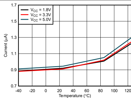
図 6-6. 10Hz I_{CCAVG} と温度との関係
