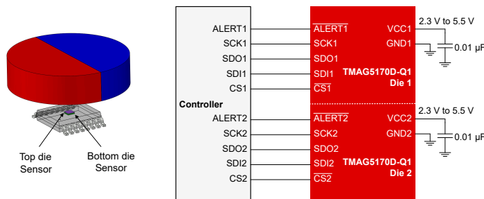
アプリケーションのブロック図
