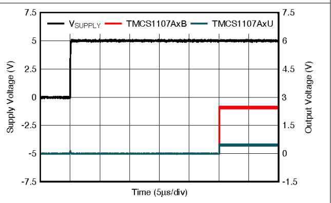
図 7-12. スタートアップ過渡応答
