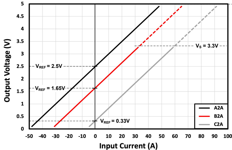
図 8-3. TMCS11xx2A の出力電圧と入力電流との関係
