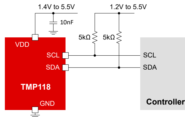
概略回路図
