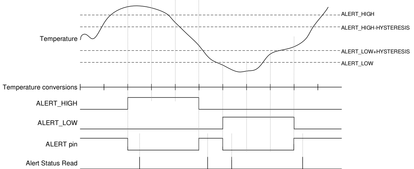
図 8-18. コンパレータ モードのタイミング図
