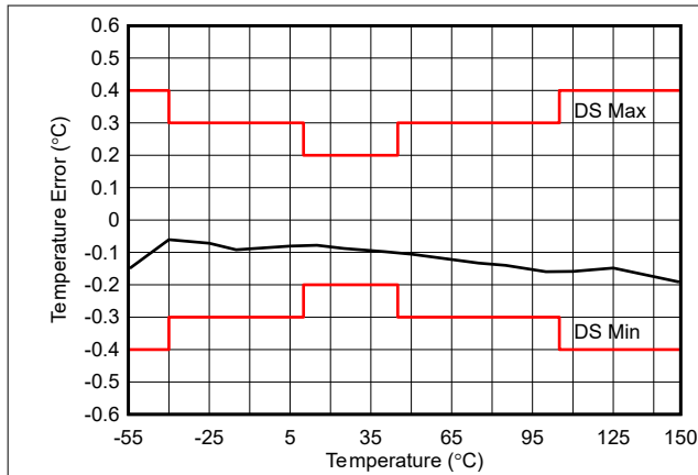
図 7-7. 温度誤差と温度との関係 (NGR パッケージ)
