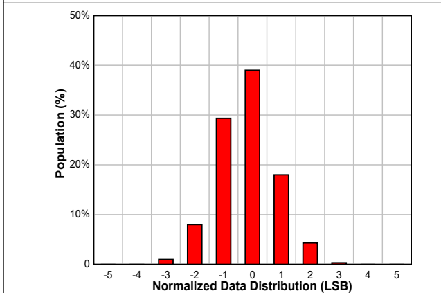
図 7-11. 変換時間 5.5ms、平均化オンでのデータの分散 (16 ビット・フォーマット)
