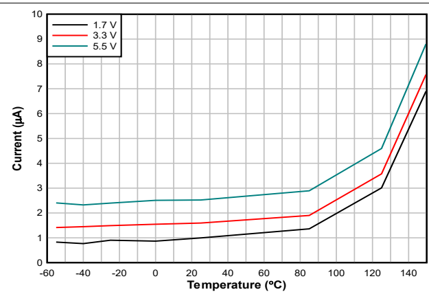
図 7-10. スタンバイ電流と温度との関係
