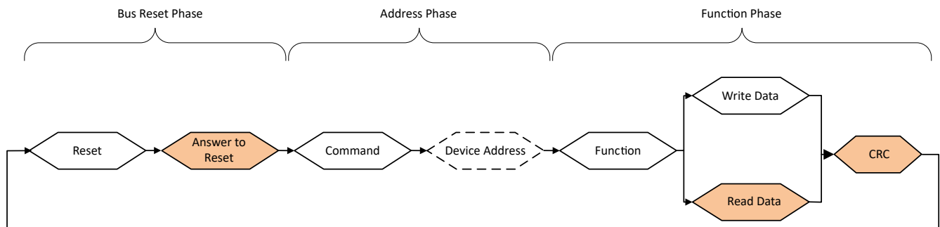
図 8-19. 1-Wire® バス通信
