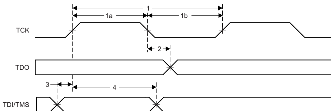
图 4-12. JTAG Timing
