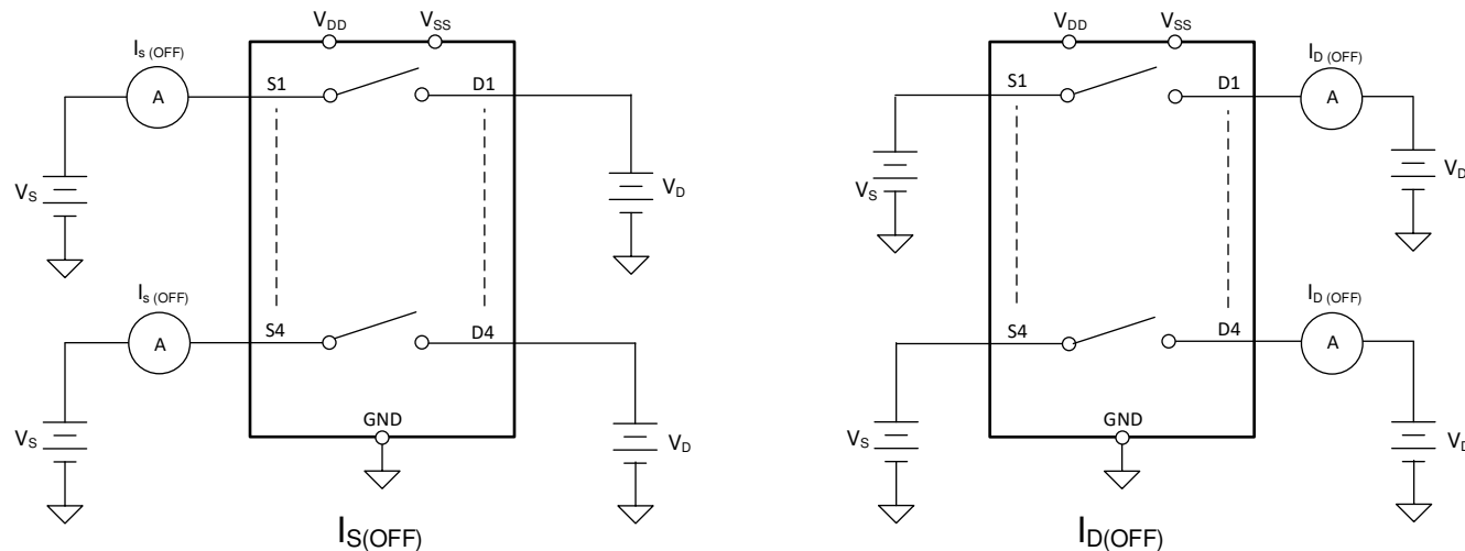
図 16-2. オフ リーク測定時の構成
