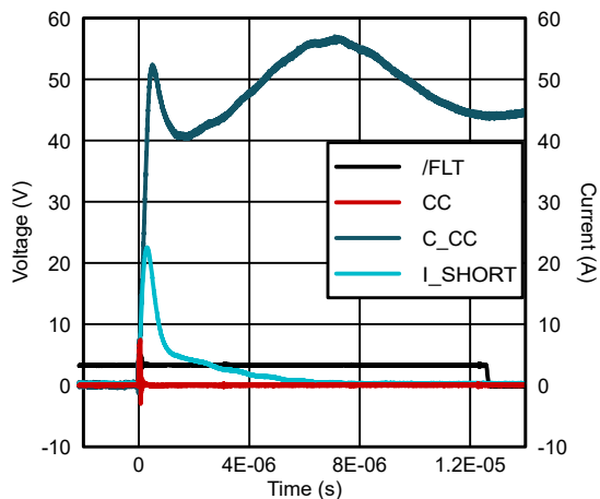
図 5-5. CC の V_{BUS} 短絡保護 48V
