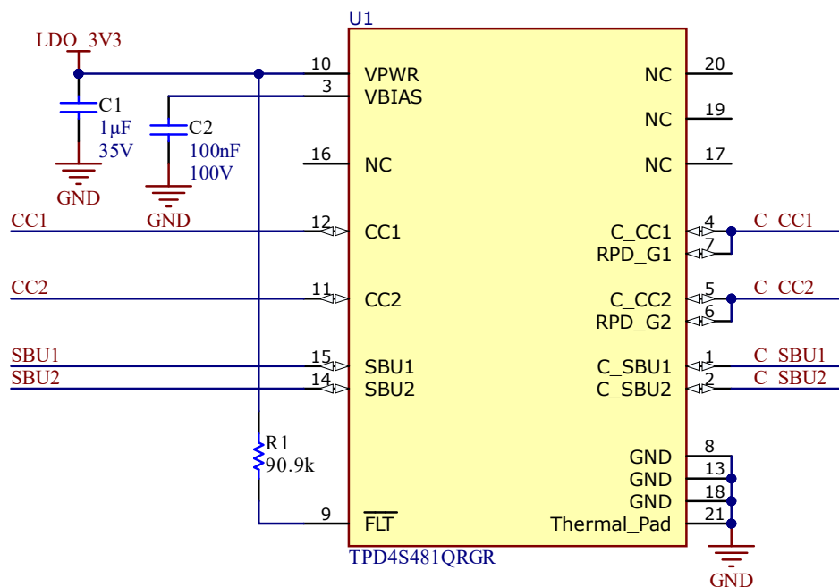
図 7-2. TPD4S481-Q1 デッドバッテリー
