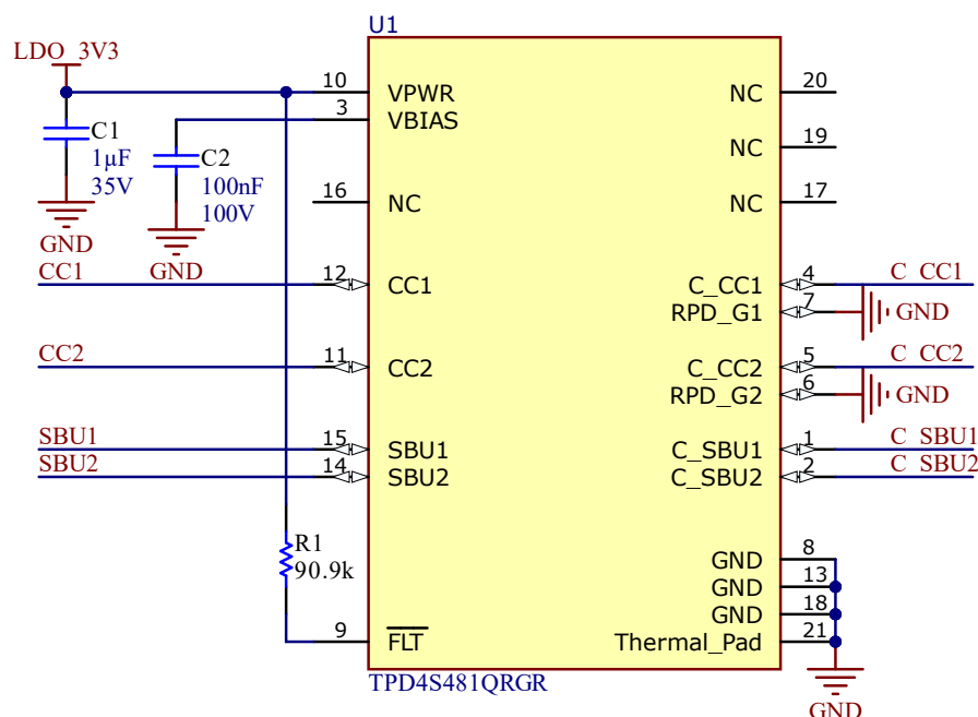
図 7-1. TPD4S481-Q1 デッドバッテリーなし
