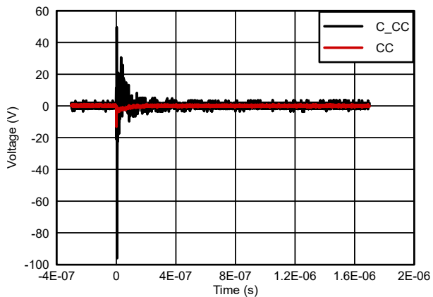
図 5-7. CC IEC 61000-4-2 -8kV 応答波形
