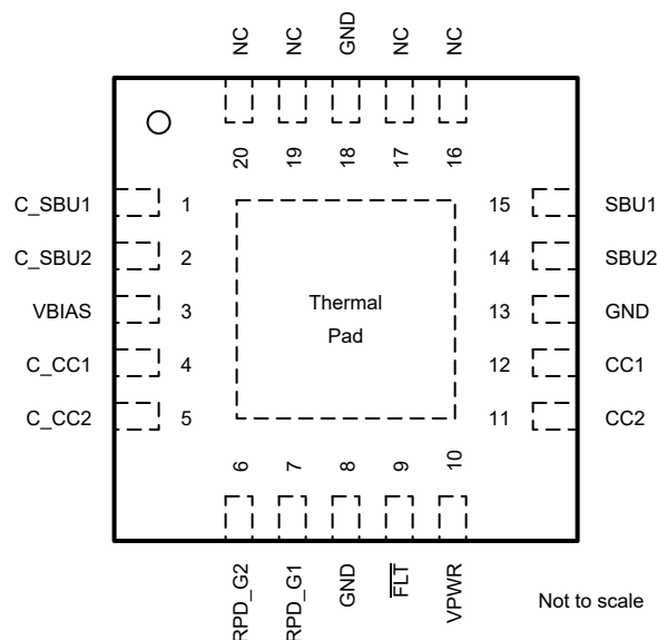
図 4-1. TPD4S481-Q1 RGR パッケージ、20 ピン QFN
