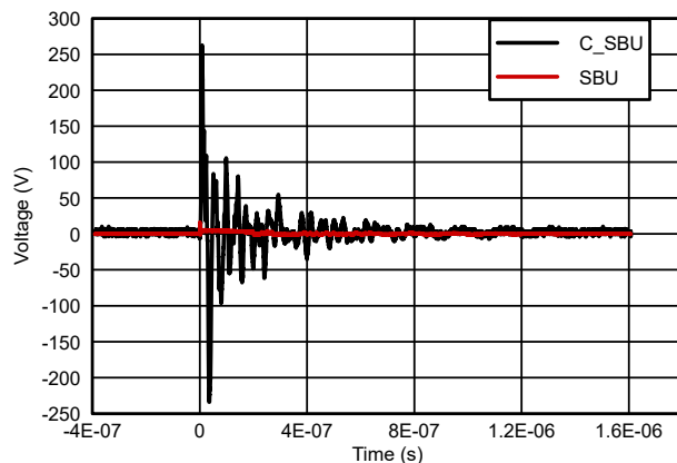
図 5-3. SBU IEC 61000-4-2 4kV 応答波形
