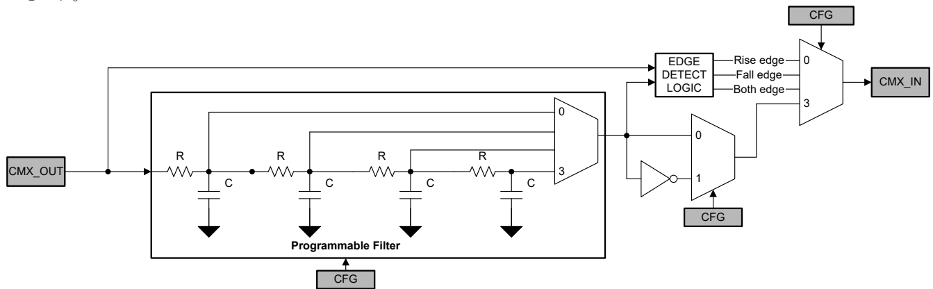
図 7-22. プログラム可能なフィルタ / エッジ検出器のブロック図
