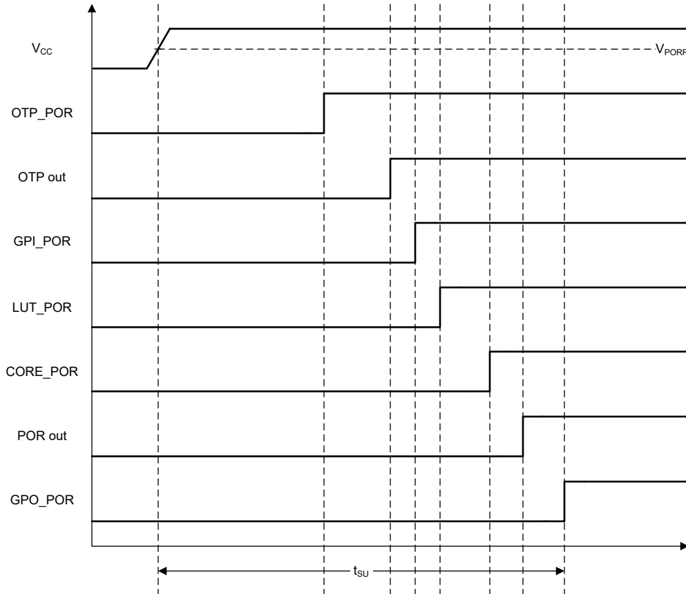
図 7-65. POR シーケンス
