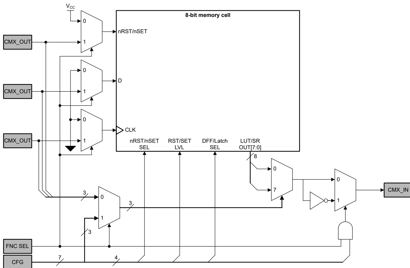
図 7-7. 3 ビット LUT または DFF / ラッチ (nRST/nSET 付き) または 8 ビット SISO シフトレジスタのブロック図
