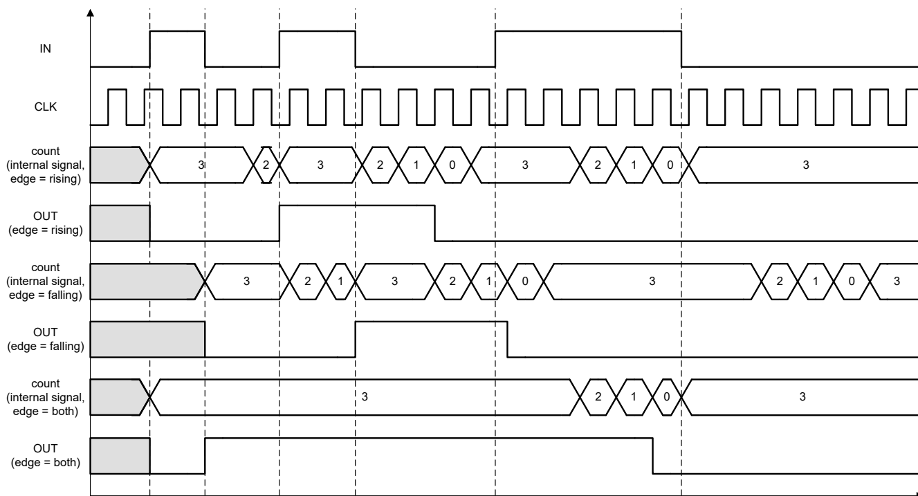
図 7-19. 周波数コンパレータの出力タイミングの例 (データ = 3)
