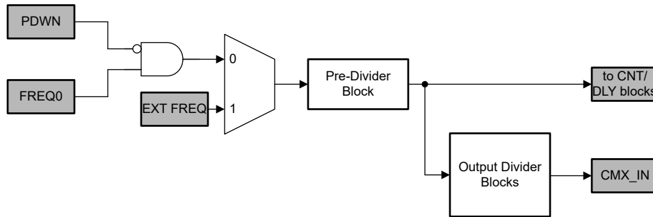
図 7-49. 固定周波数発振器のブロック図
