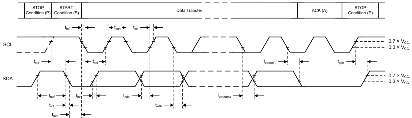
図 7-51. I 2 C 読み出し/書き込みのタイミング図
