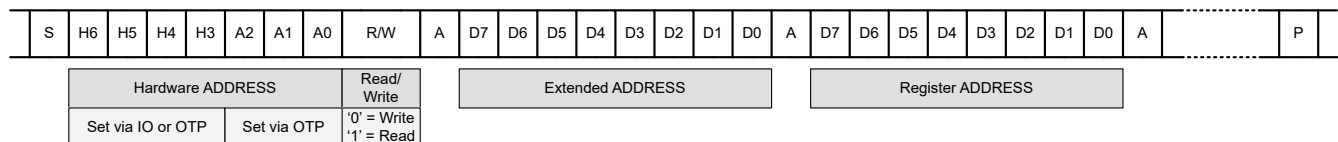
図 7-52. TPLD I 2 C のフレームとフォーマット
