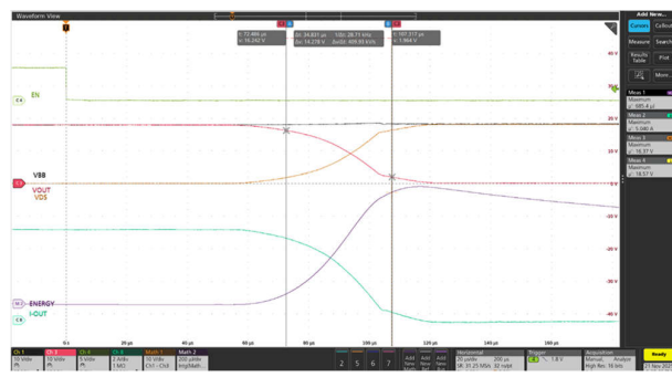
VBB = 13.5V I OUT1 = 5A T AMB = 25°C V EN = 5V ~ 0V
