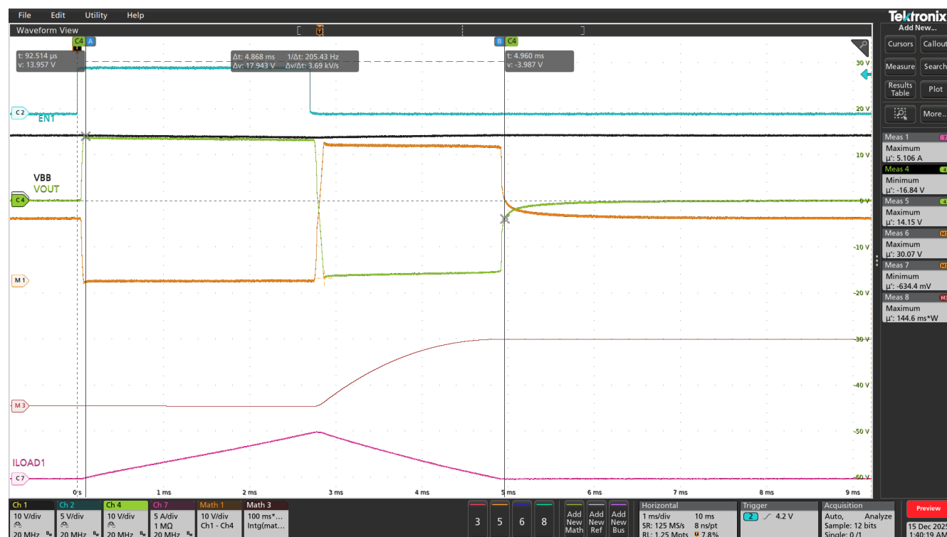
図 8-25. 5mH 誘導性負荷ドライブ ( V_{BB} = 13.5V 、 T_{AMB} = 125^{\circ}C )
