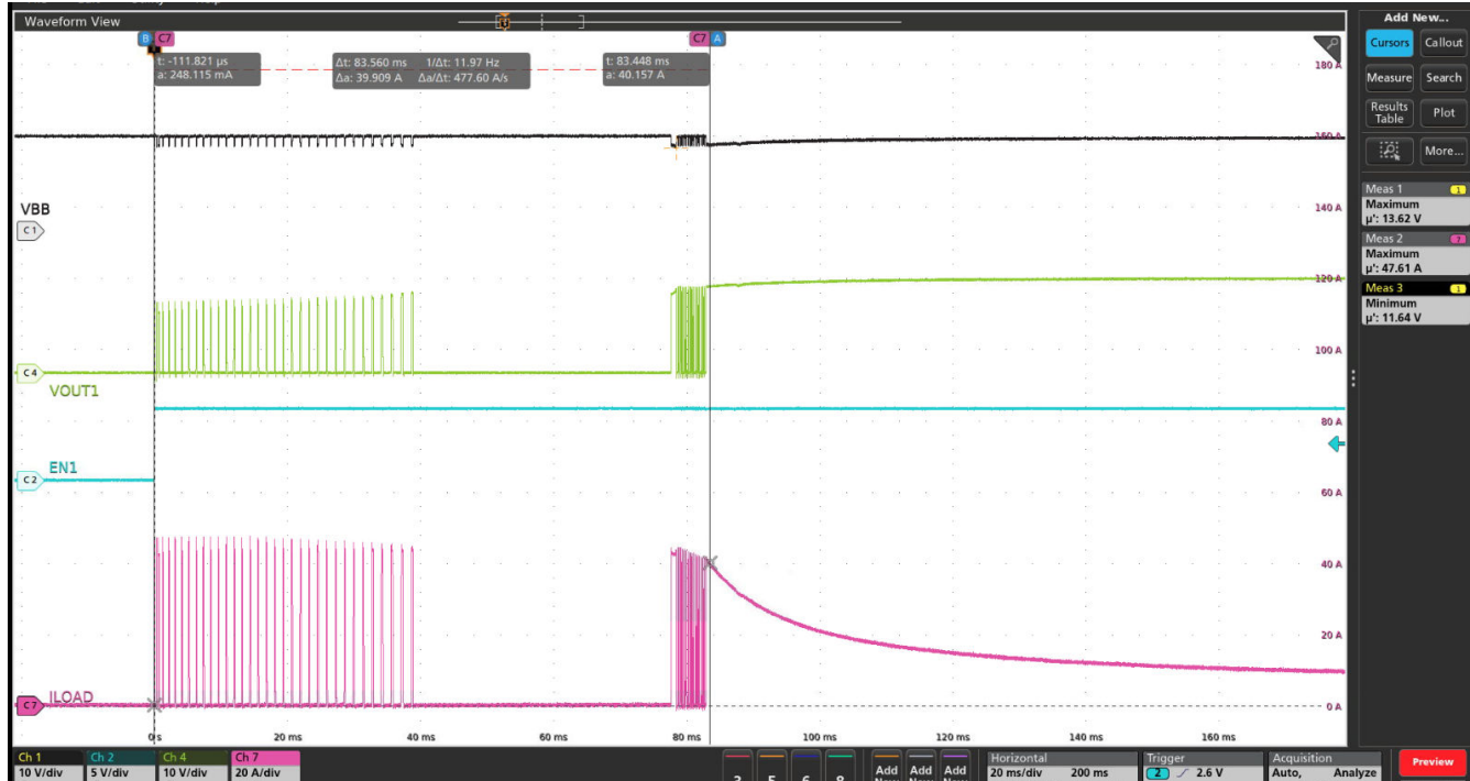
図 8-34. 13.5V VBB 条件下における TPS1HC04-Q1 シングルチャネル使用時の 100W バルブ充電特性、 T_A (device) = 25°C、 T_A (bulb) = -40°C、ILIM = GND
