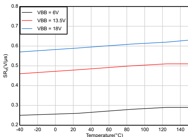
図 6-9. VOUT 立ち上がりスループレート ( SR_R ) と温度 (P、M パージョン) との関係
