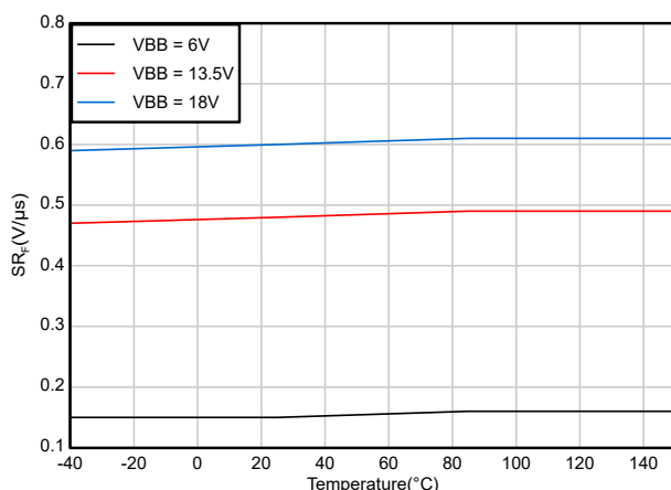
図 6-10. VOUT 立ち下がりスループレート ( SR_F ) と温度 (P、M パージョン) との関係
