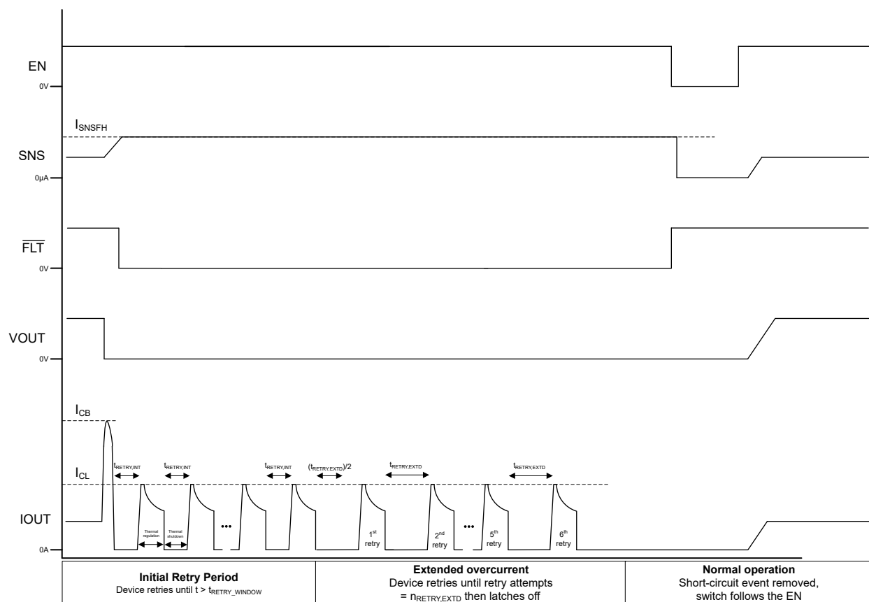
図 8-20. サーマルレギュレーションによるホット短絡後の再試行動作
