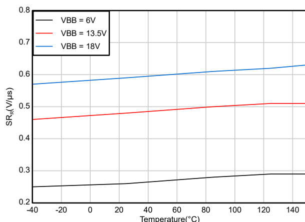
図 6-9. VOUT 立ち上がりスループレート ( SR_R ) と温度 (P、M バージョン) との関係
