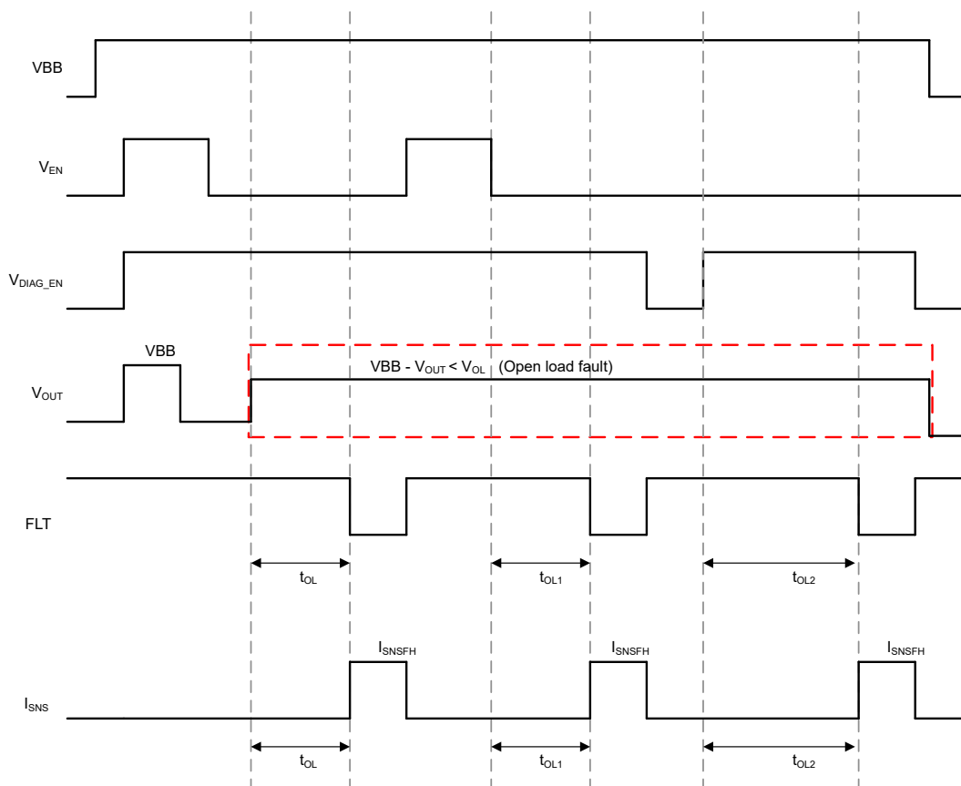
図 8-32. オフ状態での開放負荷検出
