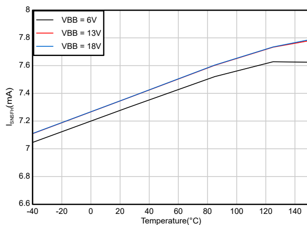
図 6-6. I_{\text{SNS}} 故障 High レベル電流と温度との関係
