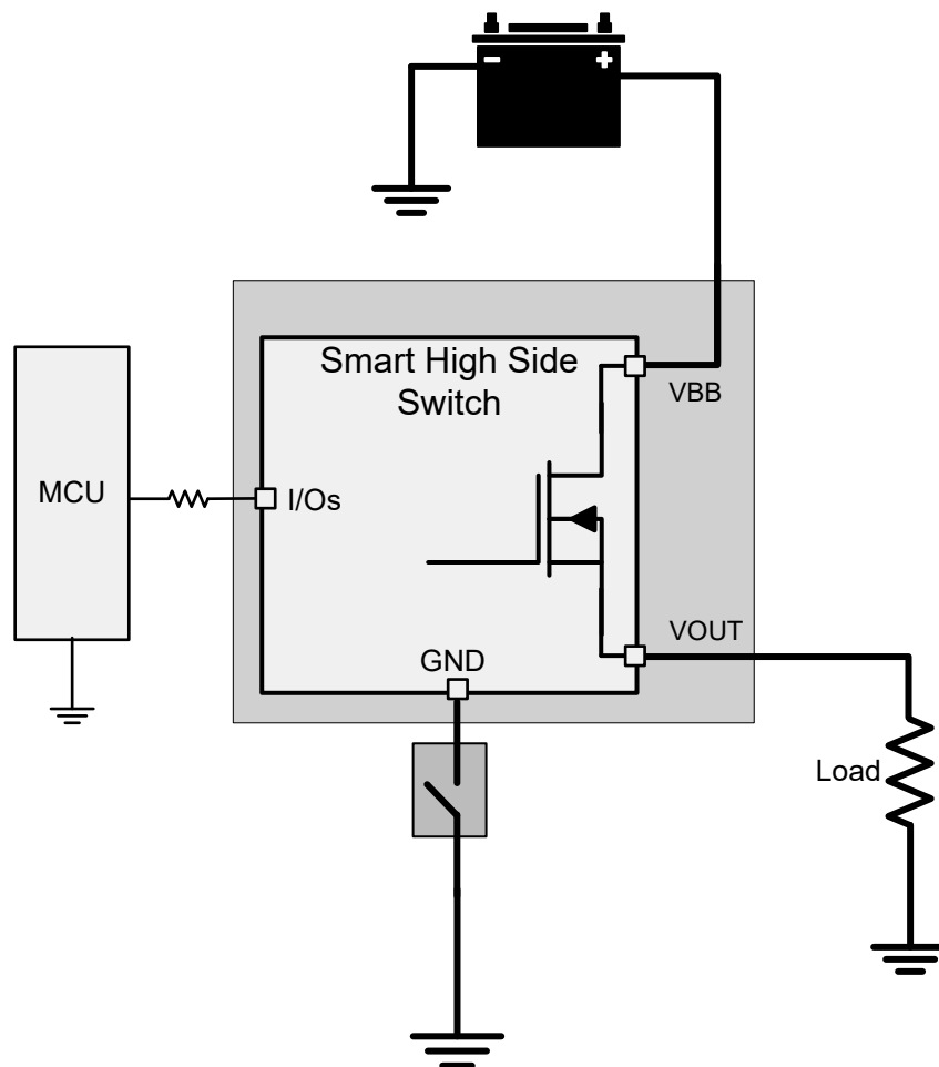
図 8-35. デバイスの GND 喪失
