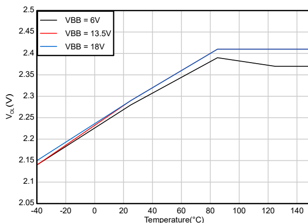
図 6-18. 開放負荷検出電圧 ( V_{OL} ) と温度との関係
