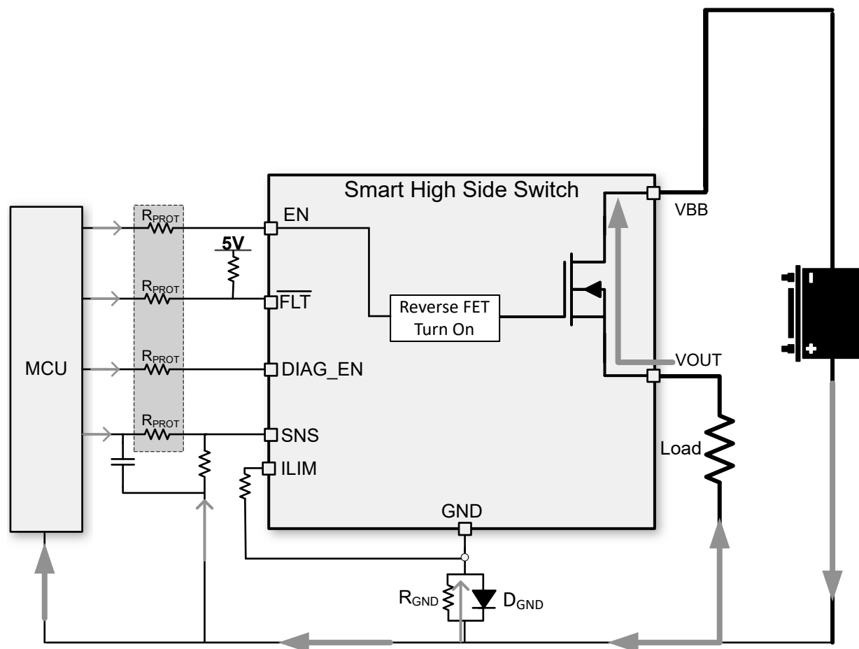
図 8-40. マイコン I/O 保護
