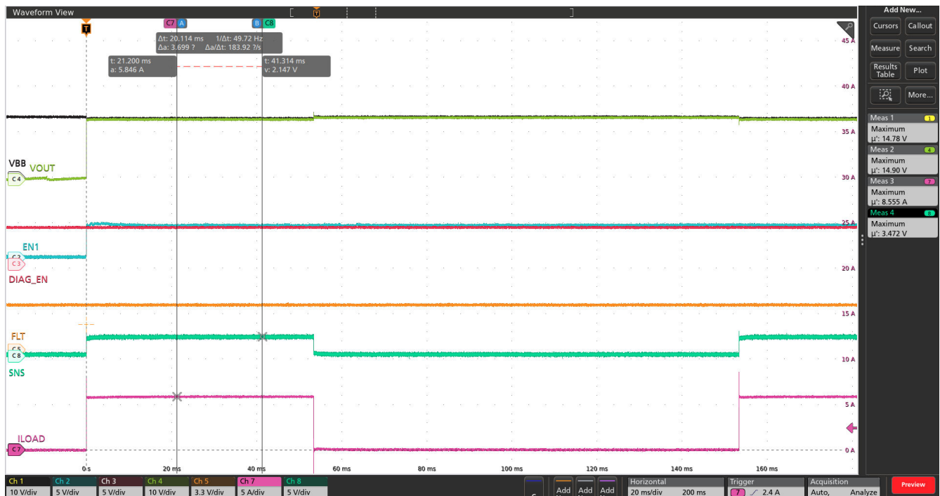
図 8-4. 負荷電流変化時の SNS ピン電圧 ( R_{SNS} = 1k\Omega )
