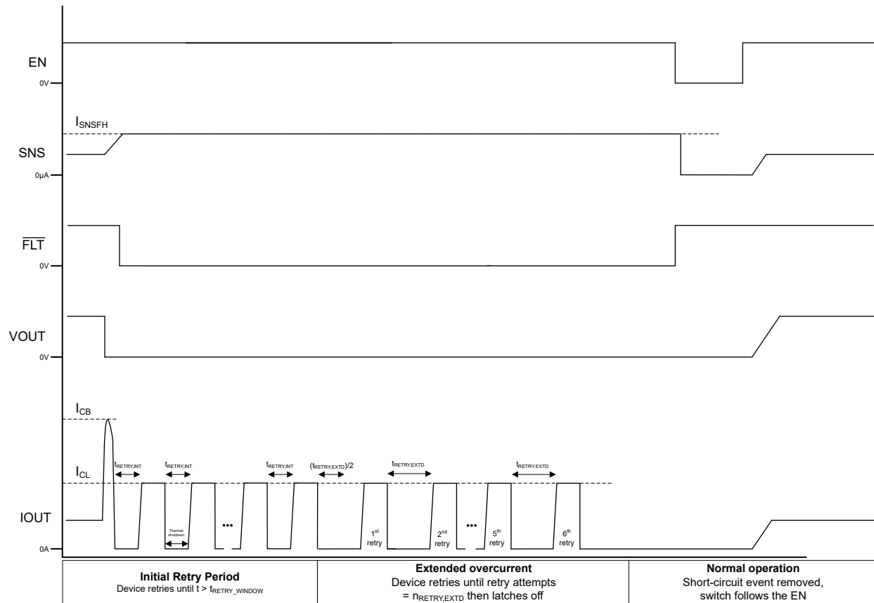
図 8-21. サーマルレギュレーションなしでのホット短絡後の再試行動作
