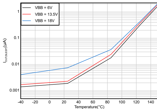
図 6-3. 出力リーク電流 ( I_{\text{OUT(SLEEP)}} ) と温度との関係
