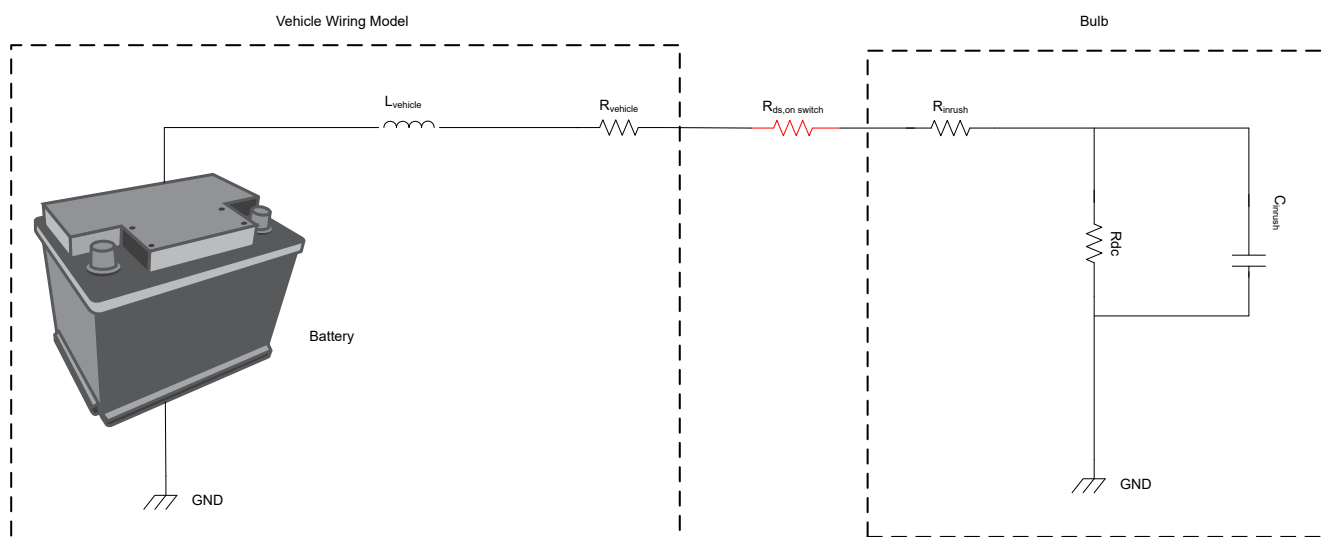
図 8-31. 簡略化した車両アーキテクチャ モデル
