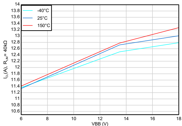
図 6-20. 電流制限レギュレーションレベル ( I_{CL} ) と VBB との関係、 R_{LIM} = 40k\Omega
