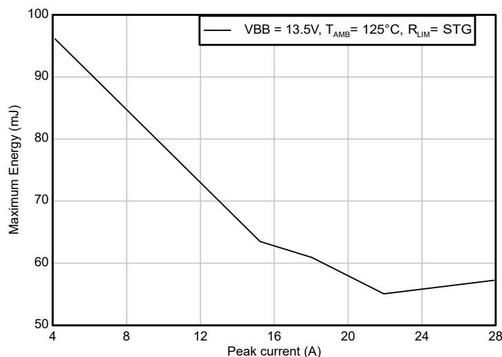
図 8-27. 誘導性スイッチオフ時の最大エネルギー吸収量とピーク電流との関係 (シングルパルス、 V_{BB} = 13.5V 、 T_{AMB} = 125^{\circ}C )
