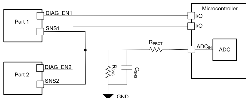
図 8-11. 複数デバイス間での SNS 多重化
