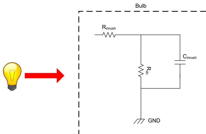
図 8-30. シンプルなバルブ モデル
