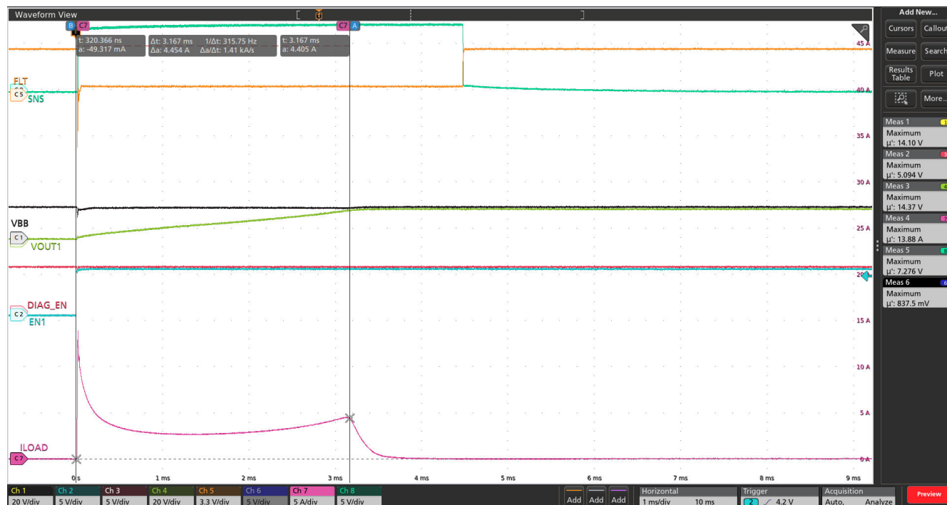
図 8-29. VBB = 13.5V、ILIM ピンをオープン、周囲温度 125°C の条件で TPS1HC08-Q1 デバイスを用いた 1mF の容量性負荷充電
