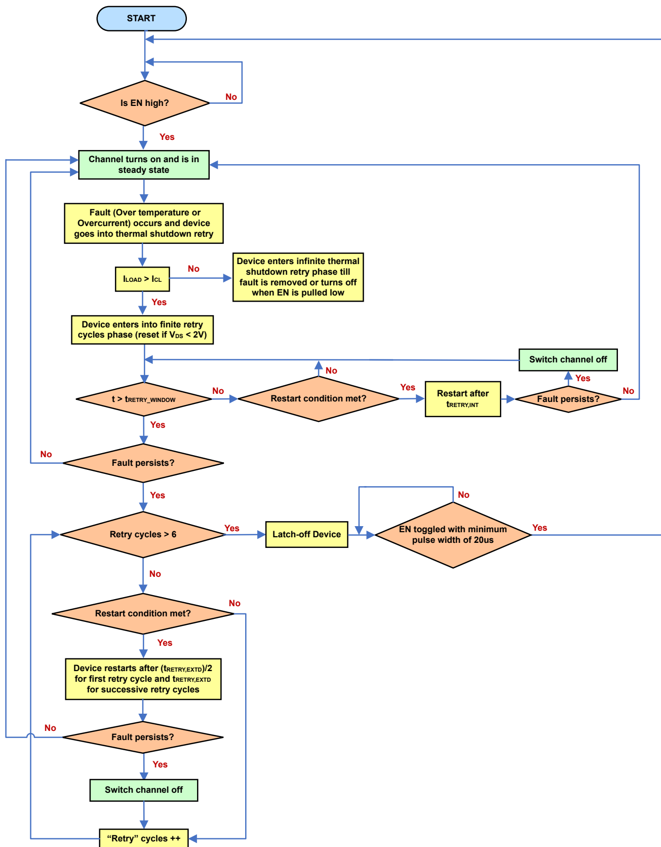
図 8-19. 再試行保護メカニズム
