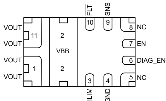
図 5-1. VAH パッケージ TPS1HC08-Q1 上面図
