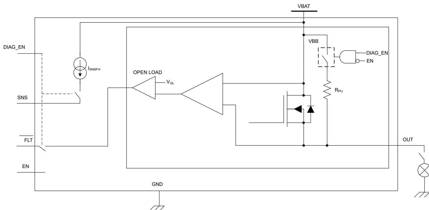
図 8-32. オフ状態での開放負荷検出
