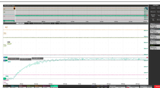
図 8-10. VBB = 13.5V、 I_{LIM} = OPEN 、 R_L = 10\Omega 、 R_{SNS} = 1k\Omega 、 T_A = 25^\circ C における 150pF C_{SNS} 使用時の SNS ピンリップル
