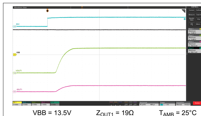
図 9-3. 抵抗性負荷でのターンオン
