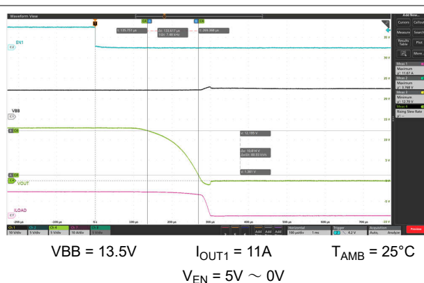
図 9-6. 立ち下がりスルーレート (D、B バージョン)
