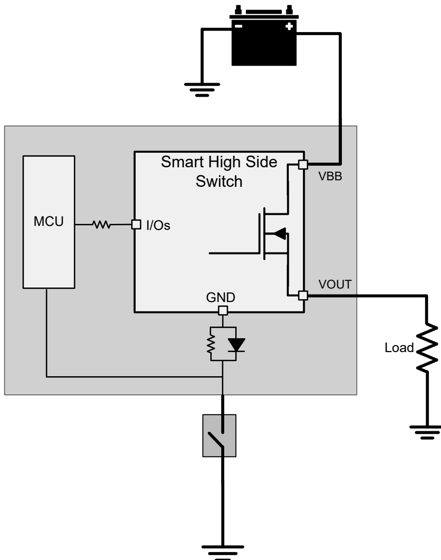
図 8-36. モジュールの GND 喪失
