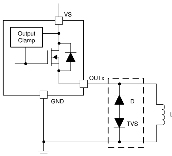
図 8-24. 外部回路による保護
