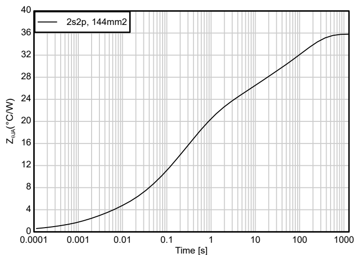
図 9-2. 露出パッド下に熱ビア 5 個を配置した EVM 2s2p PCB レイアウトにおける Z_{\Theta JA} (過渡熱インピーダンス)
