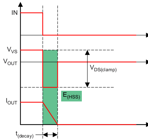
図 8-23. 誘導性負荷のスイッチングオフ図
