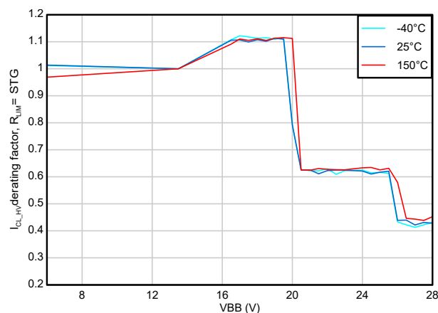
図 6-21. 電流制限ディレーティング係数 ( I_{CL\_HV} ) と VBB との関係、 R_{LIM} = \text{STG}
