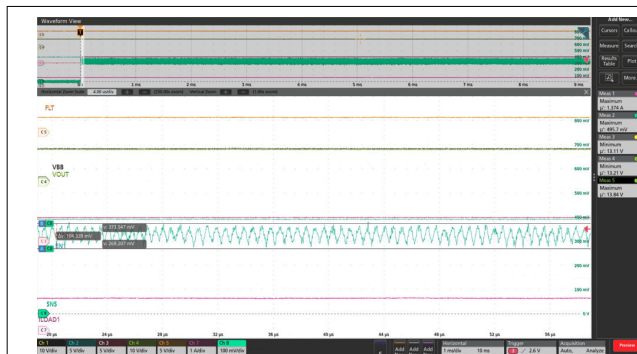
図 8-9. VBB = 13.5V、 I_{LIM} = OPEN 、 R_L = 10\Omega 、 R_{SNS} = 1k\Omega 、 T_A = 25^\circ C における C_{SNS} なし時の SNS ピンリップル
