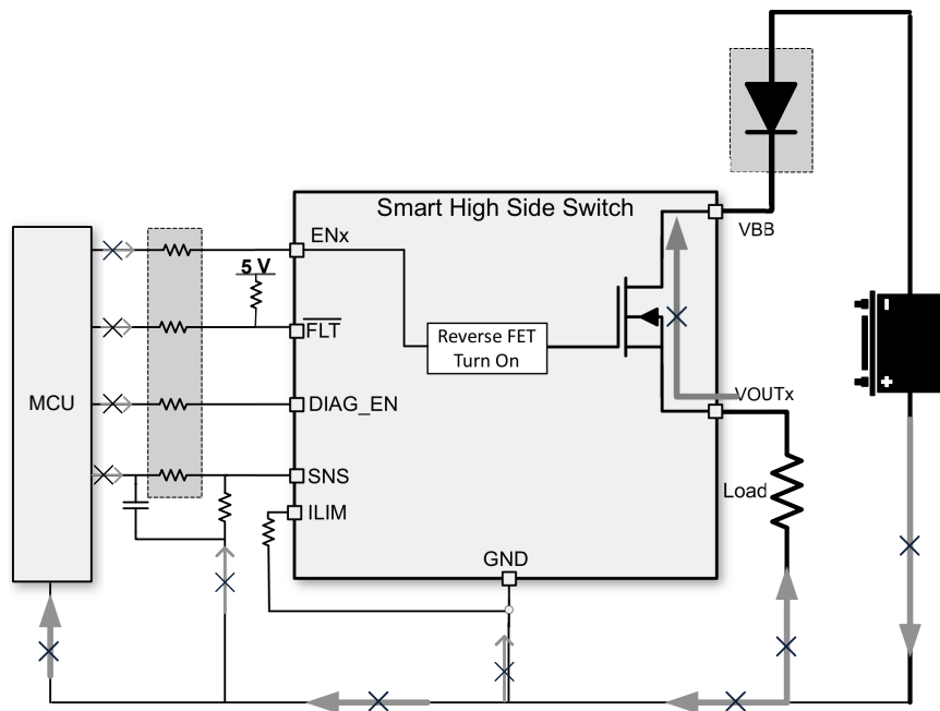
図 8-38. ブロックダイオードによる逆電流保護
