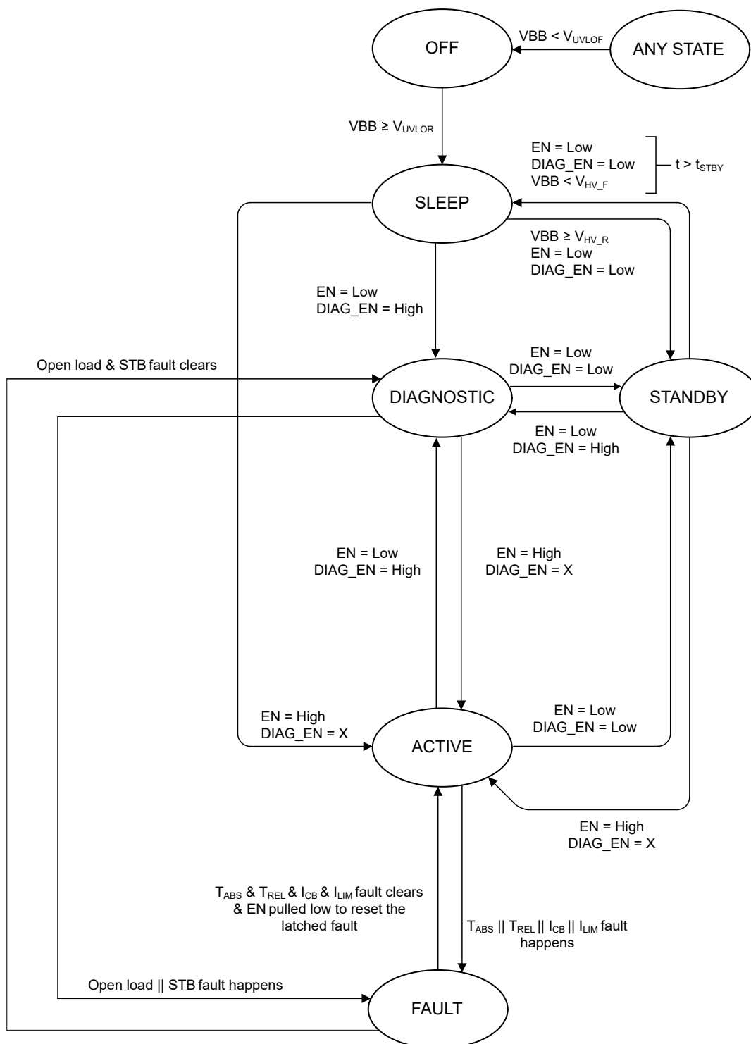
図 8-41. 状態遷移図
