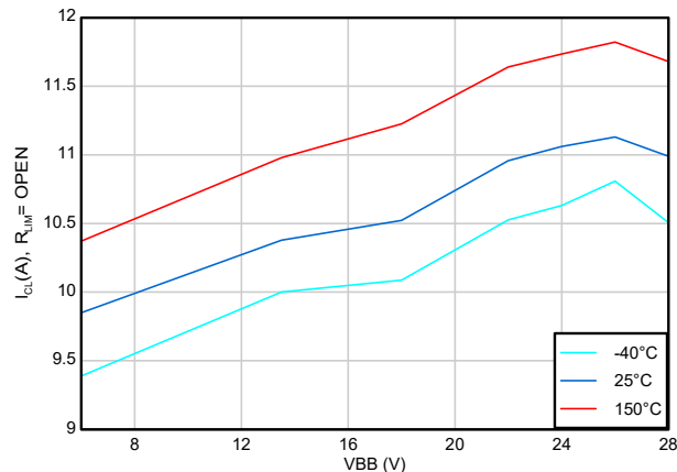
図 6-19. 電流制限レギュレーションレベル ( I_{CL} ) と VBB との関係、 R_{LIM} = \text{オープン}
