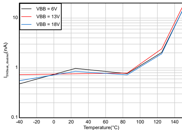
図 6-5. I_{\text{SNS}} リークエージ (Diagnostics 無効時) と温度との関係
