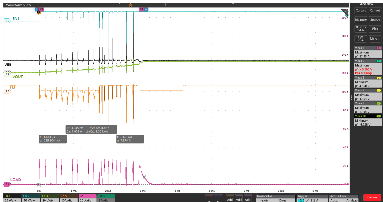
図 8-28. VBB = 13.5V、ILIM ピンをグラウンドに短絡し、周囲温度 125°C の条件で TPS1HC08-Q1 デバイスを用いた 1mF の容量性負荷充電
