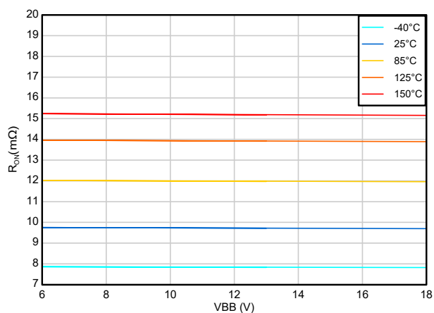
図 6-4. オン抵抗 ( R_{\text{ON}} ) と VBB との関係
