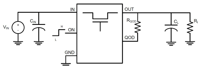
概略回路図
