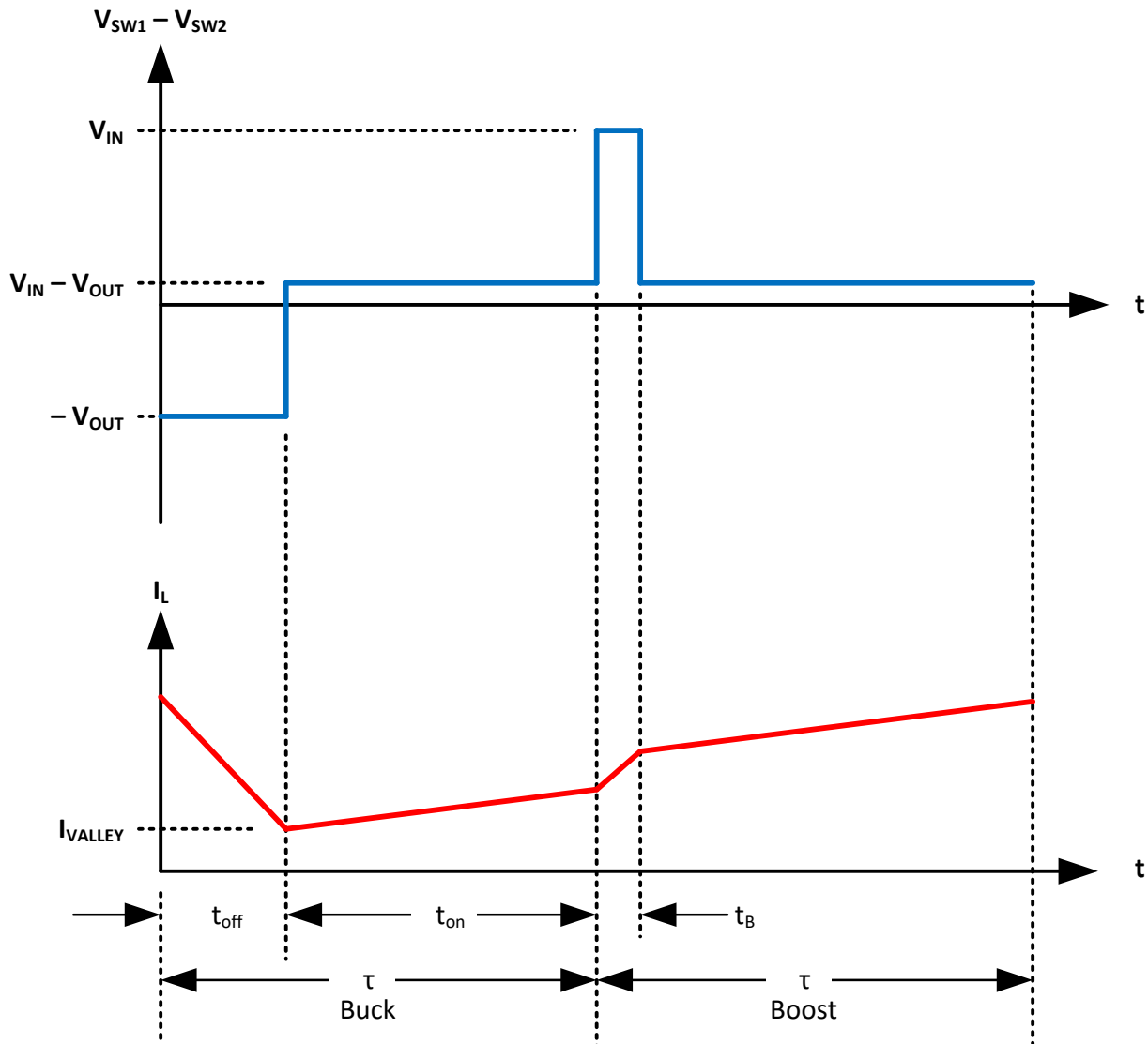
図 8-10. Buck Transition
