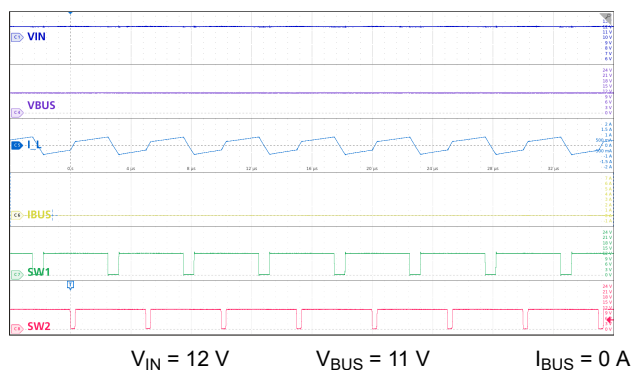
図 9-23. Buck-Boost Mode: V_{IN} \neq V_{BUS} , No Load
