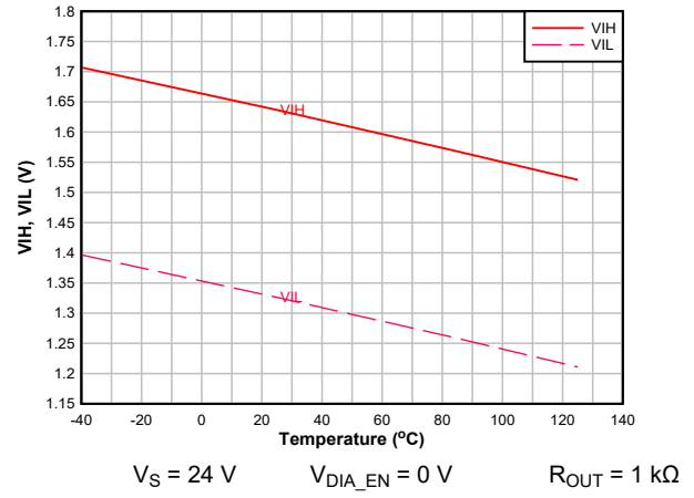
图 7-8. V_{IH} , V_{IL} vs Temperature
