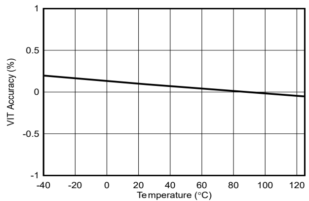
図 6-6. 固定 V_{IT} の精度と温度との関係
