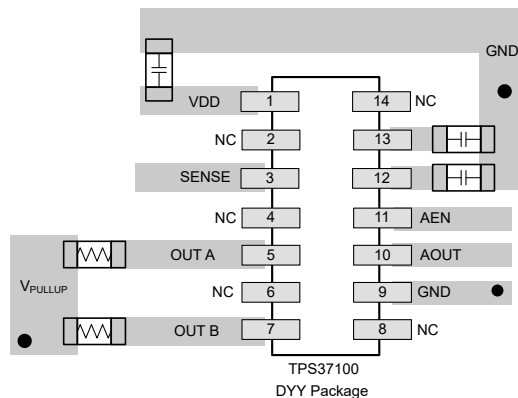
図 8-3. TPS37100 の推奨レイアウト
