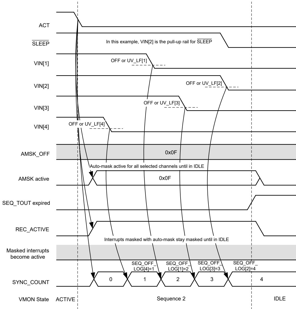
图 7-17. ACT 1→0 Transition
